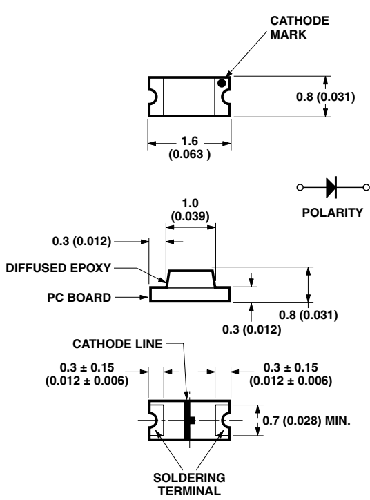
HSMB-C190
