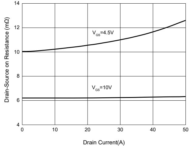
Fig. 2 - R_{DS(ON)} - I_D
